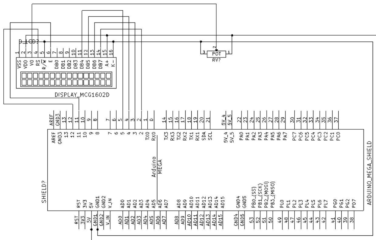
Figura 5: Esquemático Eletrônico
