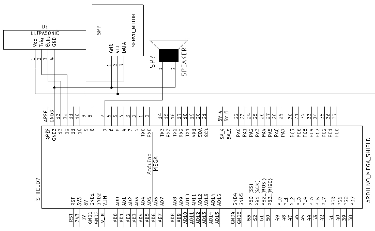
Figura 19: Esquemático Eletrônico
