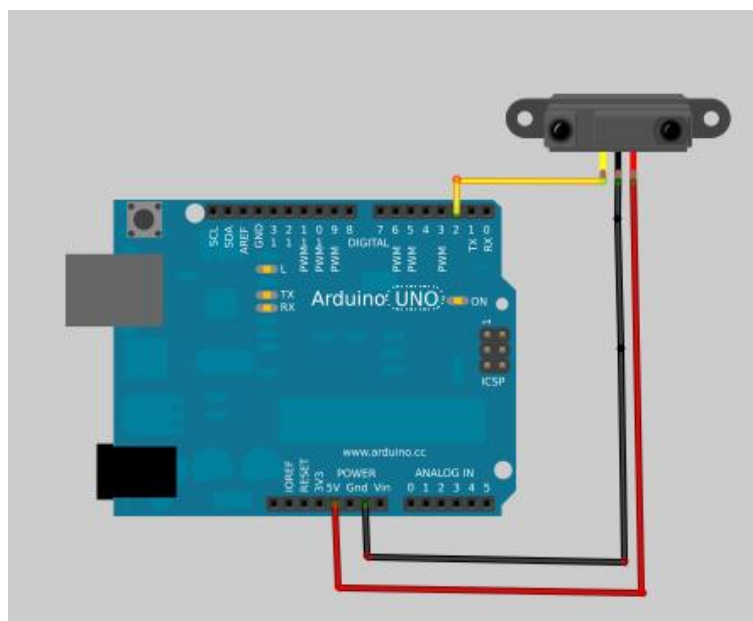
Figura 32: Sensor Infravermelho - Sharp GP2Y0A21YK0F
