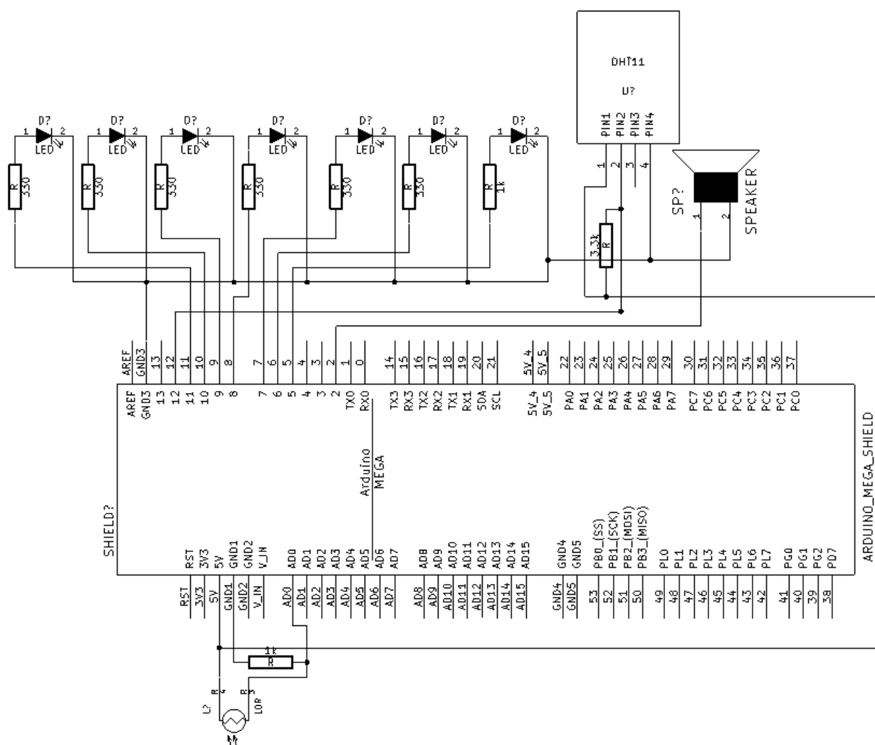
Figura 17: Esquemático Eletrônico
