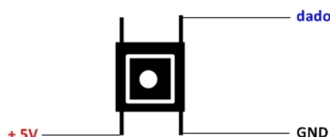
Figura 24: Pinagem do push-button de 4 terminais
