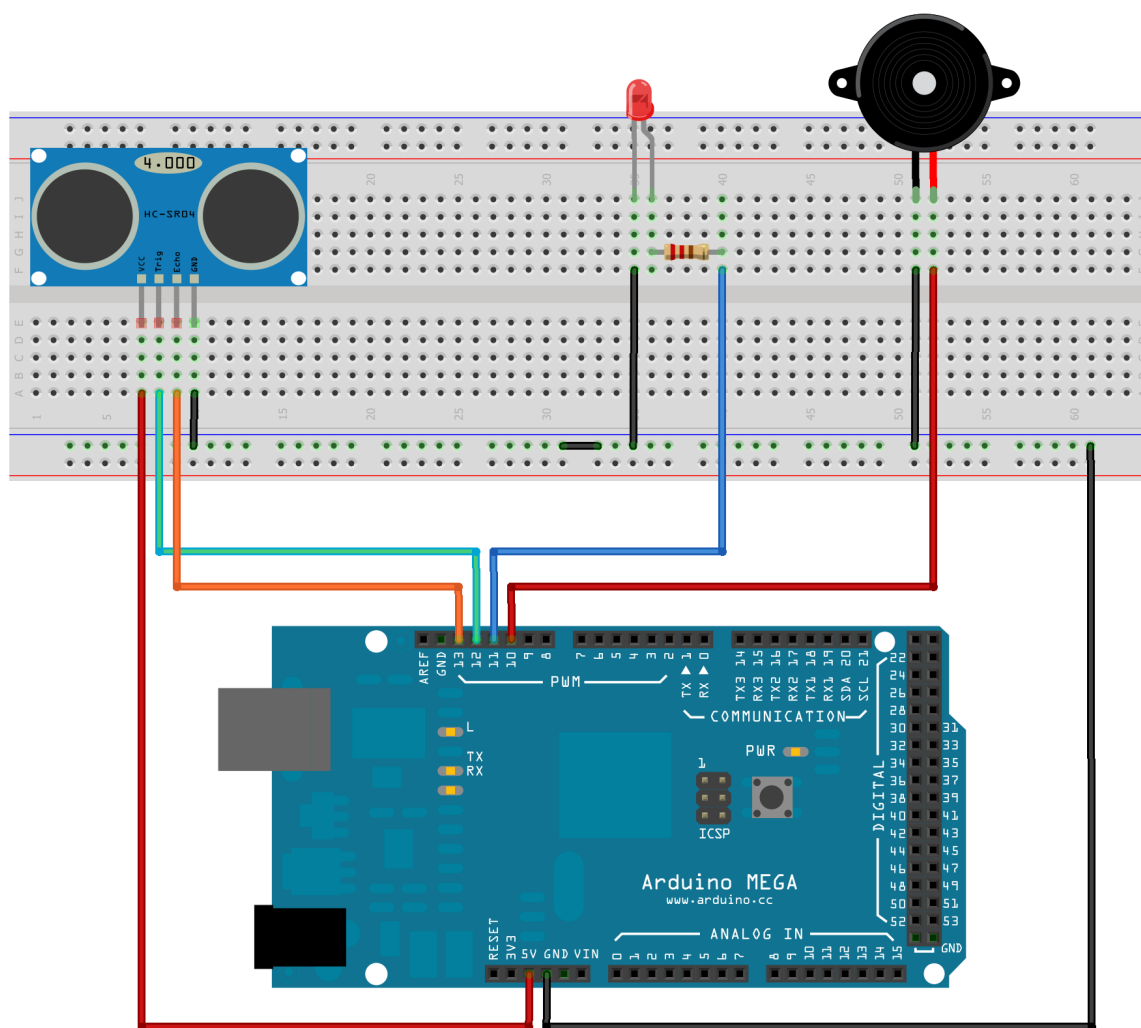
Figura 14: Montagem do Circuito
