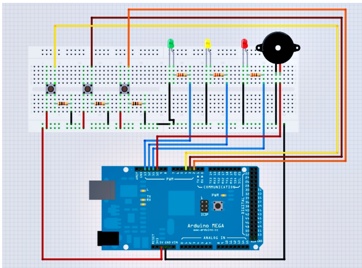
Figura 12: Montagem do Circuito
