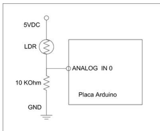
Figura 28: Esquemático do sensor de luminosidade
