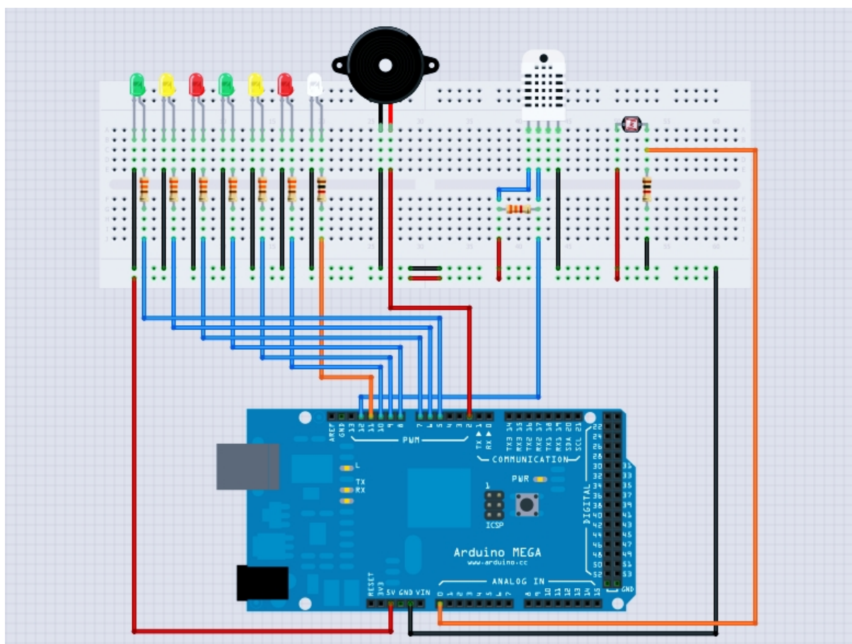
Figura 16: Montagem do Circuito
