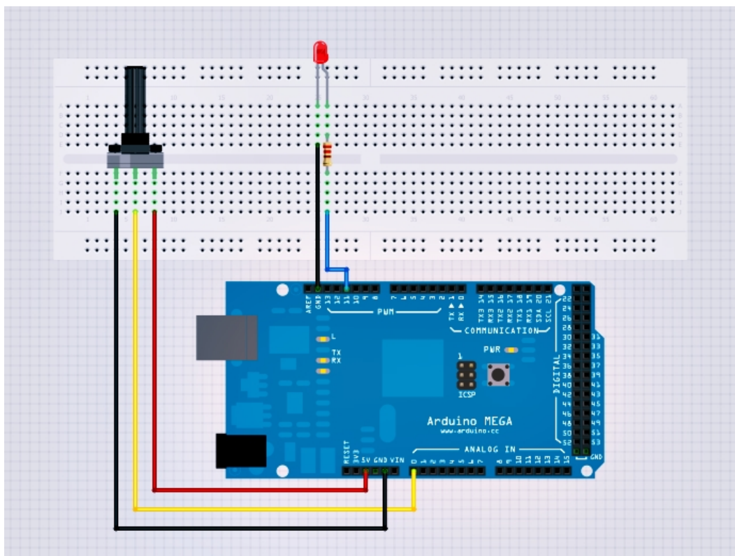
Figura 6: Montagem do Circuito
