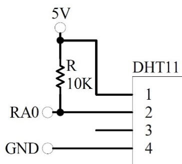
Figura 30: Sensor de temperatura e umidade DHT11 ligado a um Arduino
