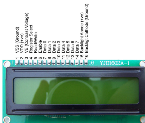
Figura 35: Descrição de cada pino de um LCD 16x2 5V
