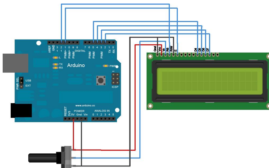
Figura 36: Pinagem de um LCD
