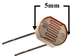
Figura 27: Sensor de Luminosidade LDR 5mm
