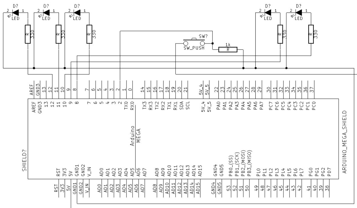
Figura 9: Esquemático Eletrônico
