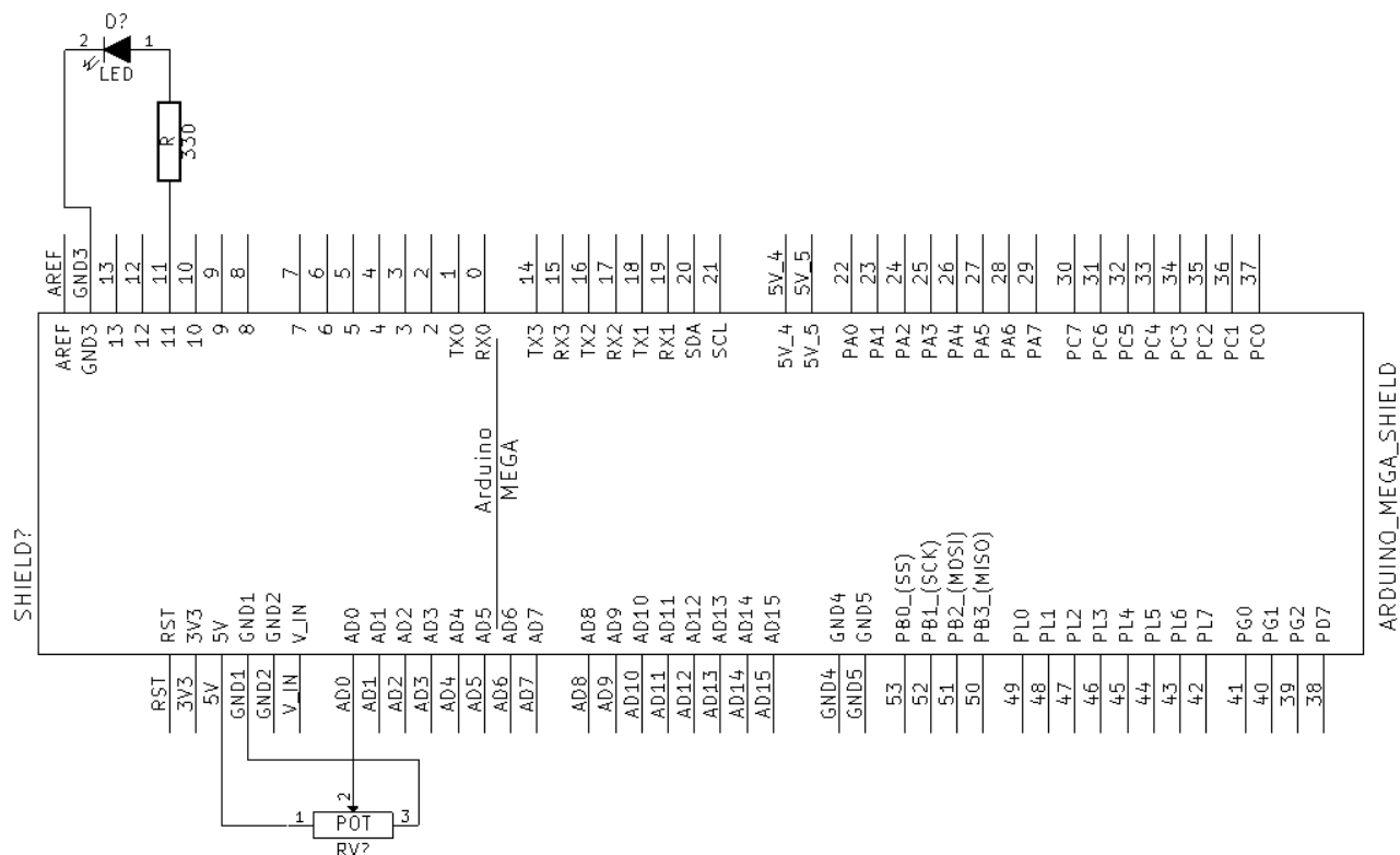
Figura 7: Esquemático Eletrônico
