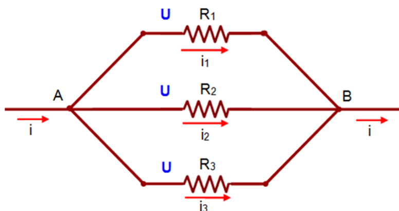
Figura 39: Associação de resistores em paralelo
