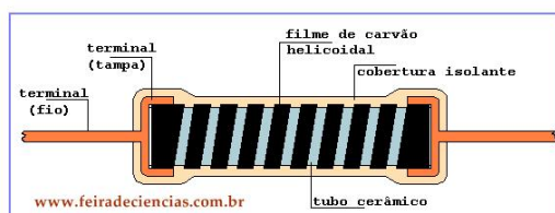
Figura 37: O resistor internamente
