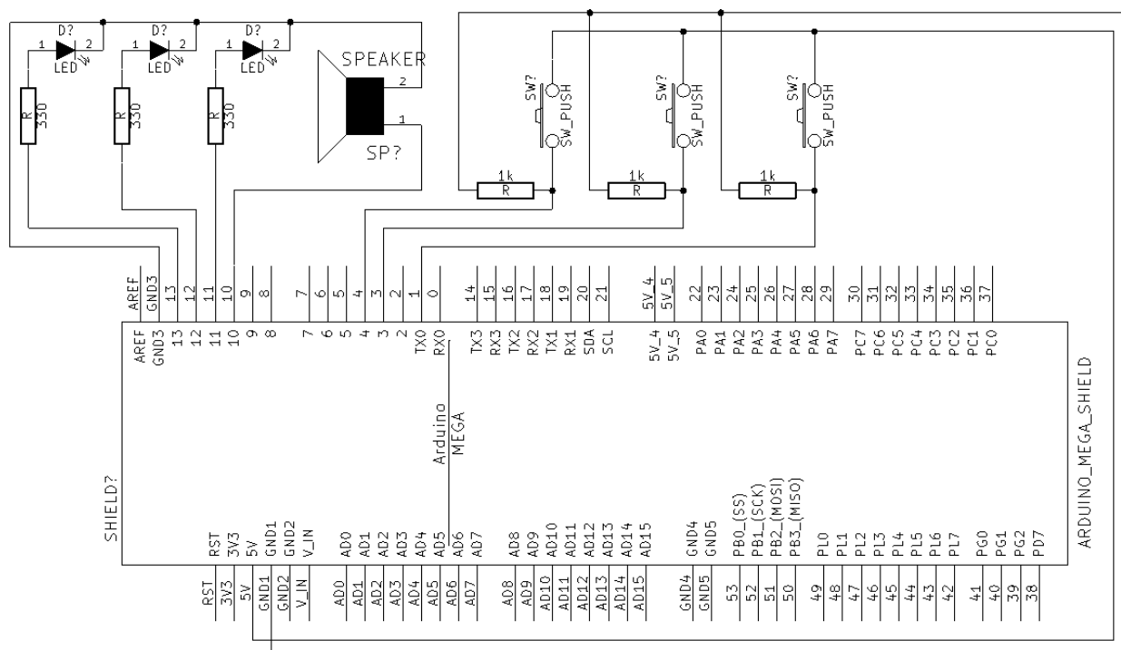
Figura 13: Esquemático Eletrônico
