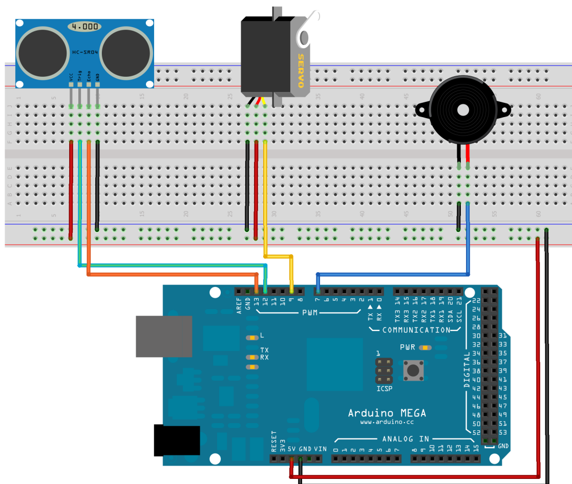
Figura 18: Montagem do Circuito
