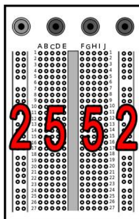
Figura 43: protoboard - divisão por matrizes
