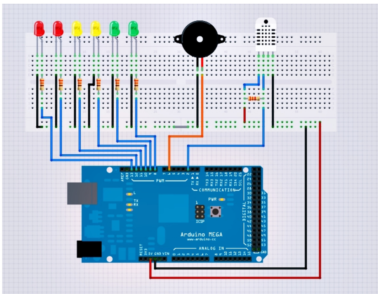
Figura 10: Montagem do Circuito
