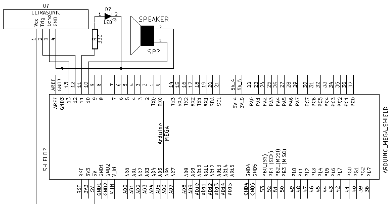
Figura 15: Esquemático Eletrônico
