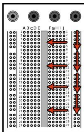
Figura 44: protoboard - transmissão nas matrizes
