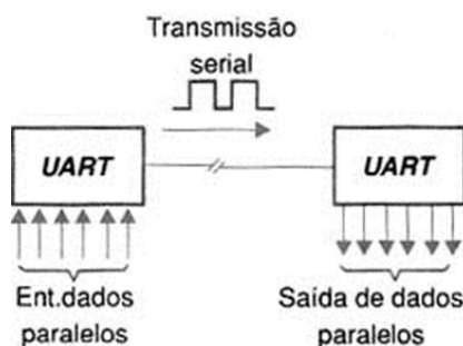
Figura 52: Funcionamento do UART
