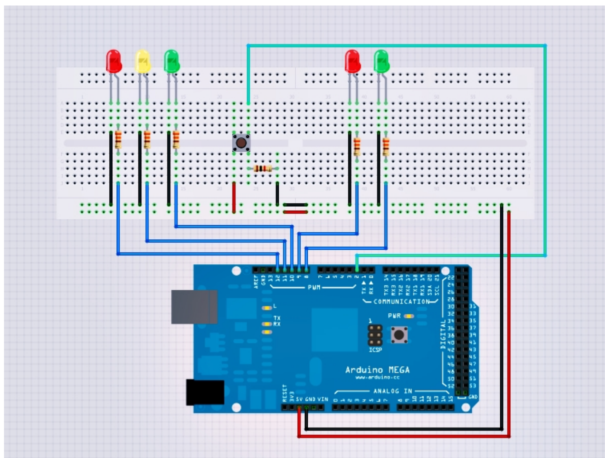
Figura 8: Montagem do Circuito
