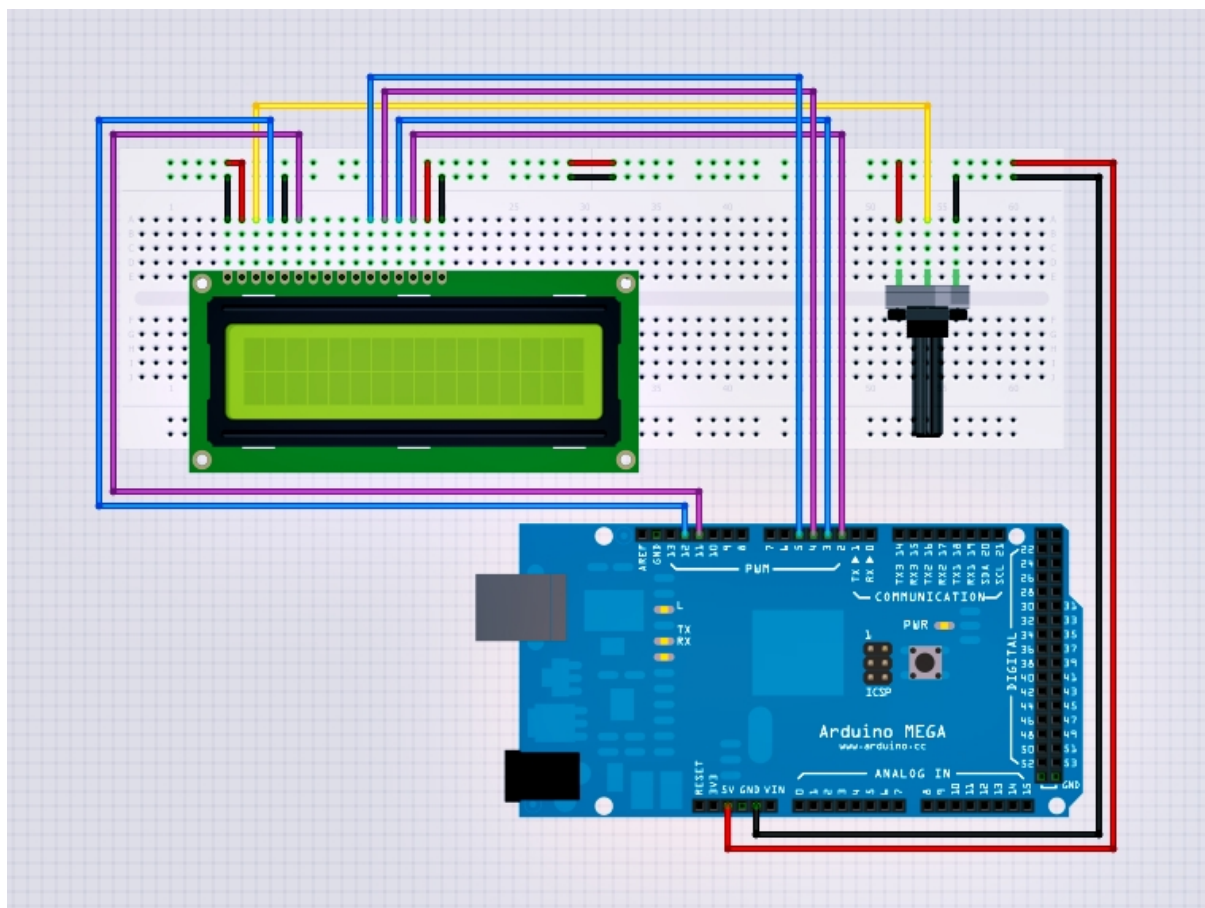
Figura 4: Montagem do Circuito
