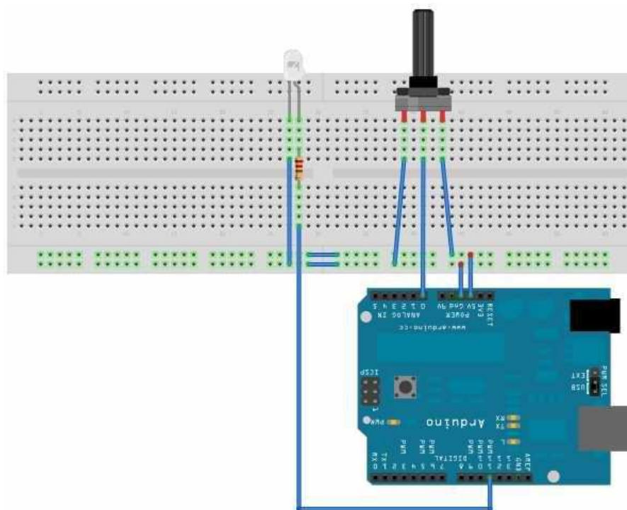
Figura 6: Montagem do Circuito
