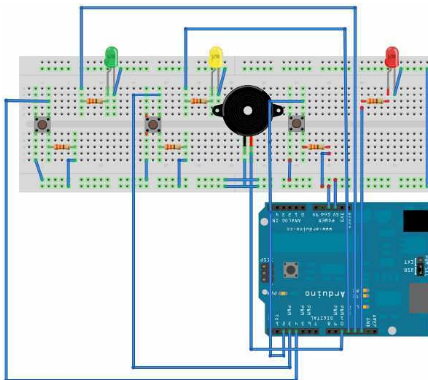
Figura 8: Montagem do Circuito
