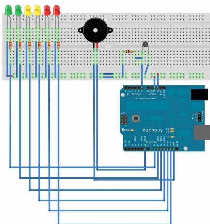
Figura 7: Montagem do Circuito
