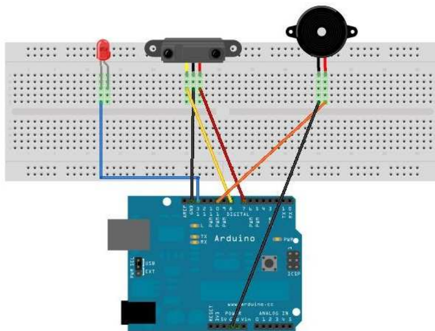
Figura 9: Montagem do Circuito
