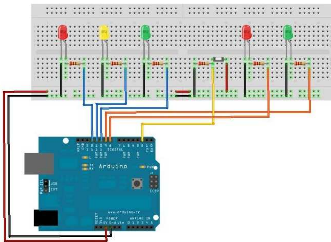
Figura 5: Montagem do Circuito
