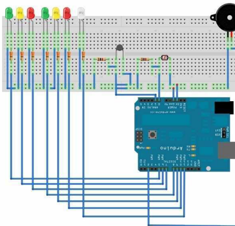
Figura 10: Montagem do Circuito
