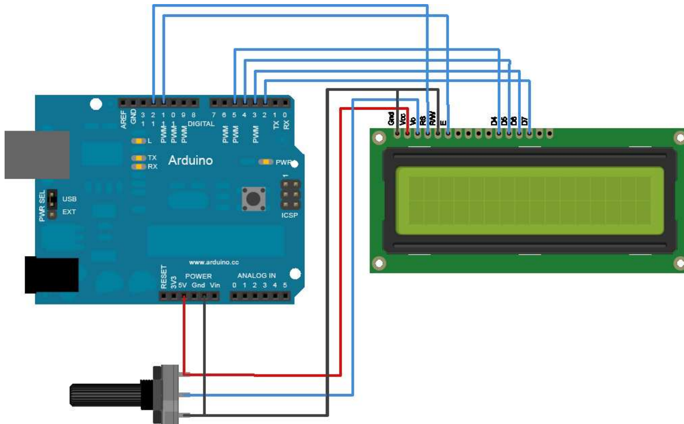
Figura 3: Exemplo usando LCD
