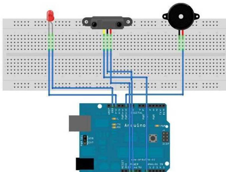
Figura 9: Montagem do Circuito
