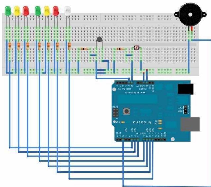
Figura 10: Montagem do Circuito
