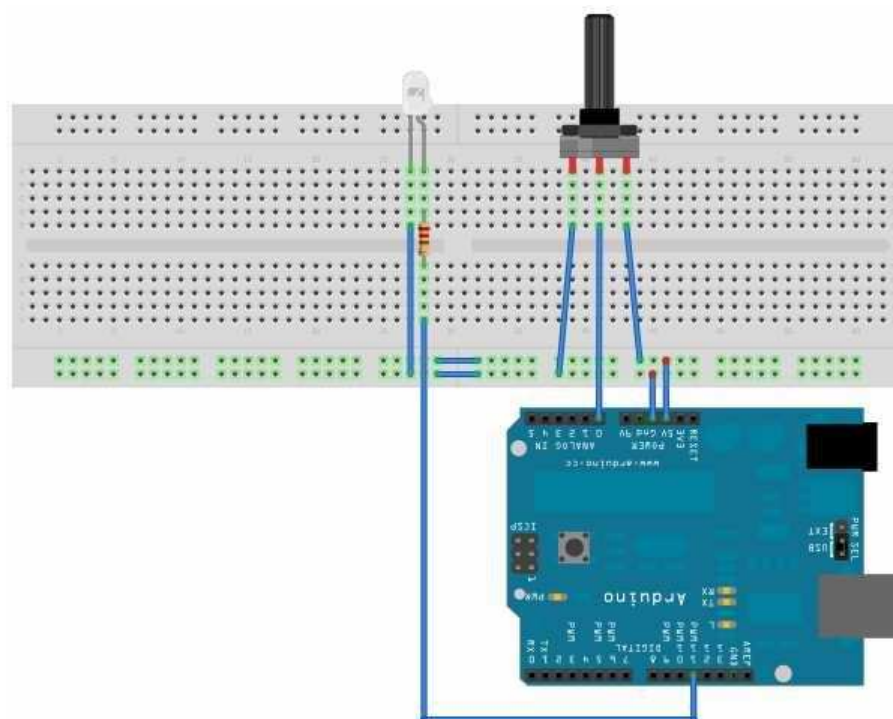
Figura 5: Montagem do Circuito
