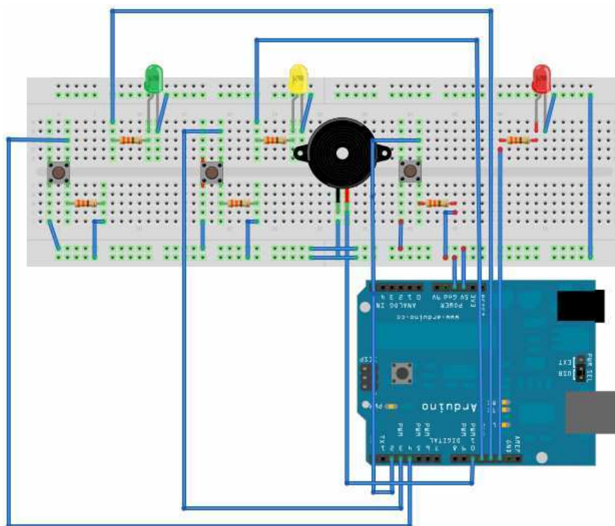
Figura 8: Montagem do Circuito
