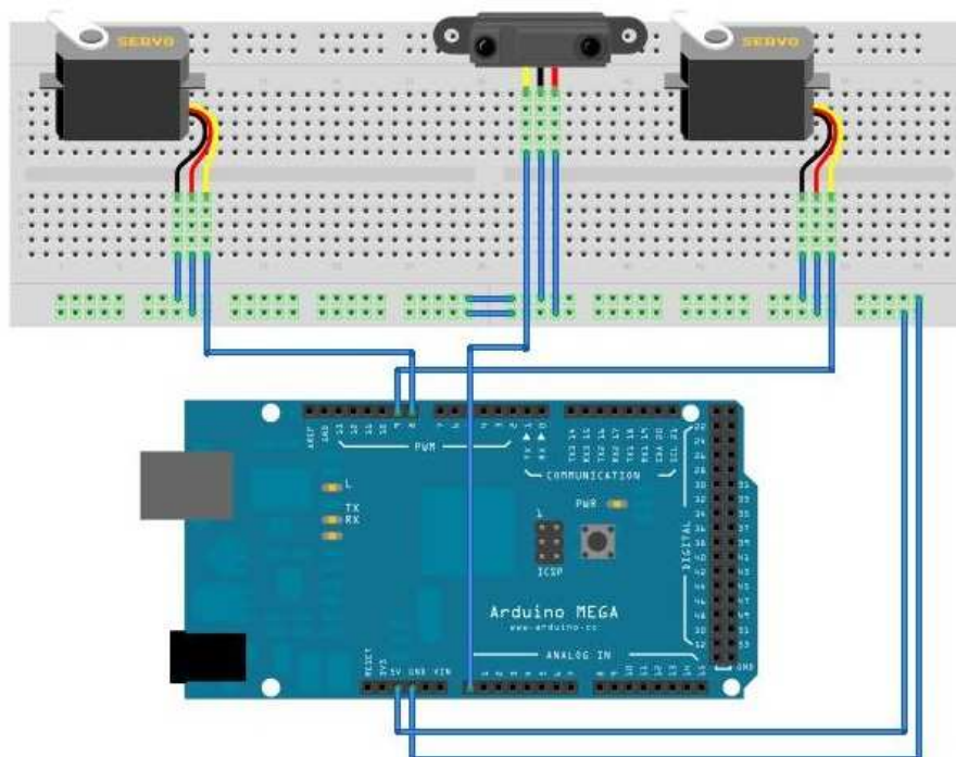
Figura 11: Montagem do Circuito
