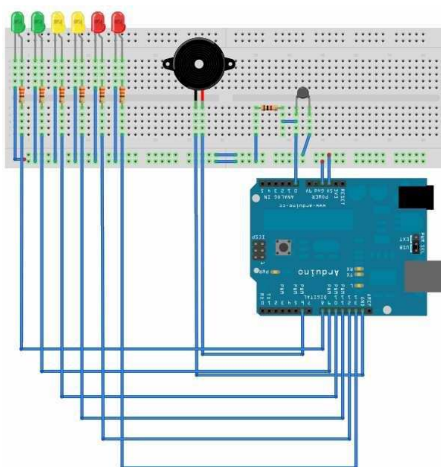
Figura 7: Montagem do Circuito
